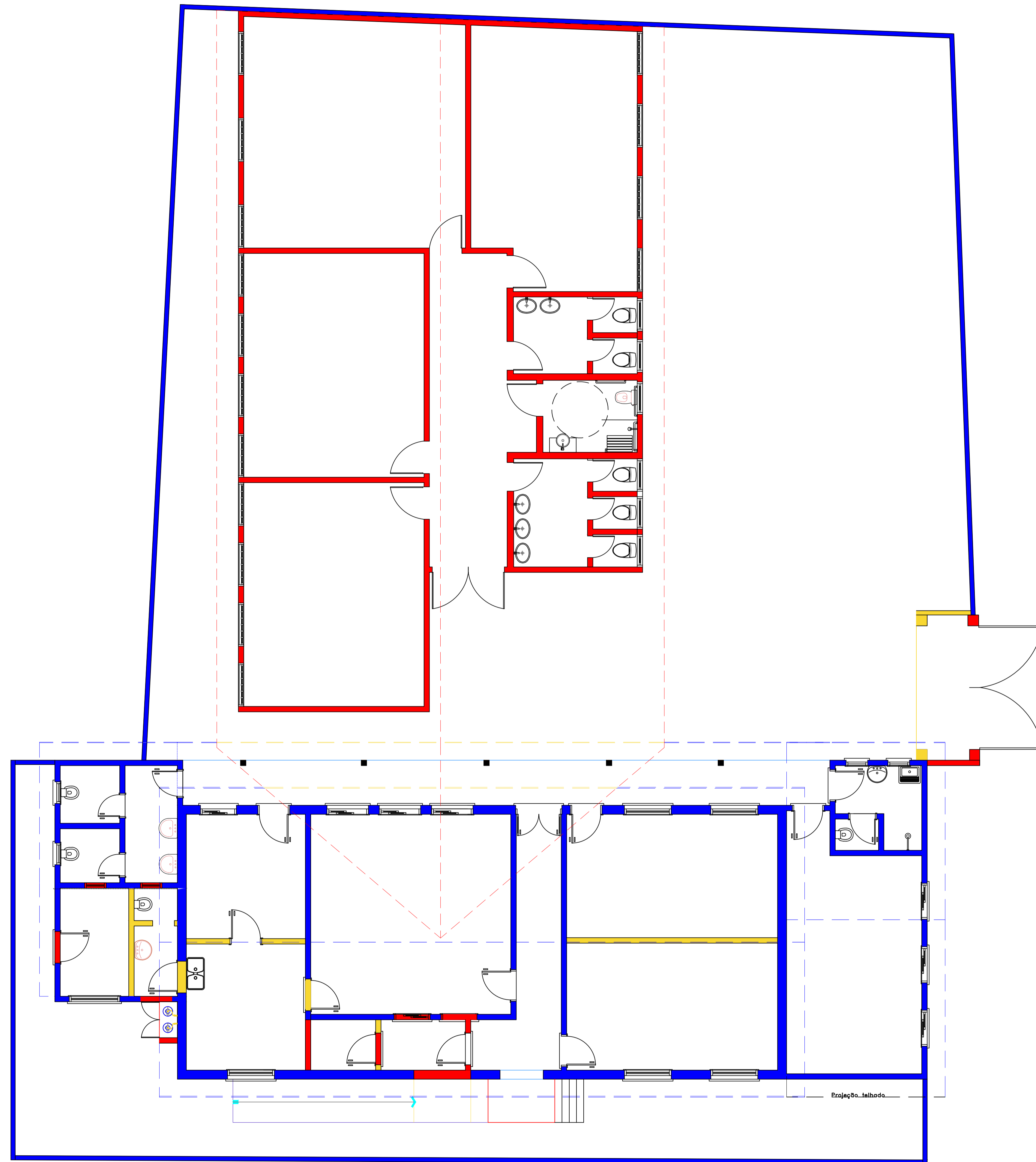
PLANTA BAIXA DE INTERVENÇÕES Esc: 1/75
