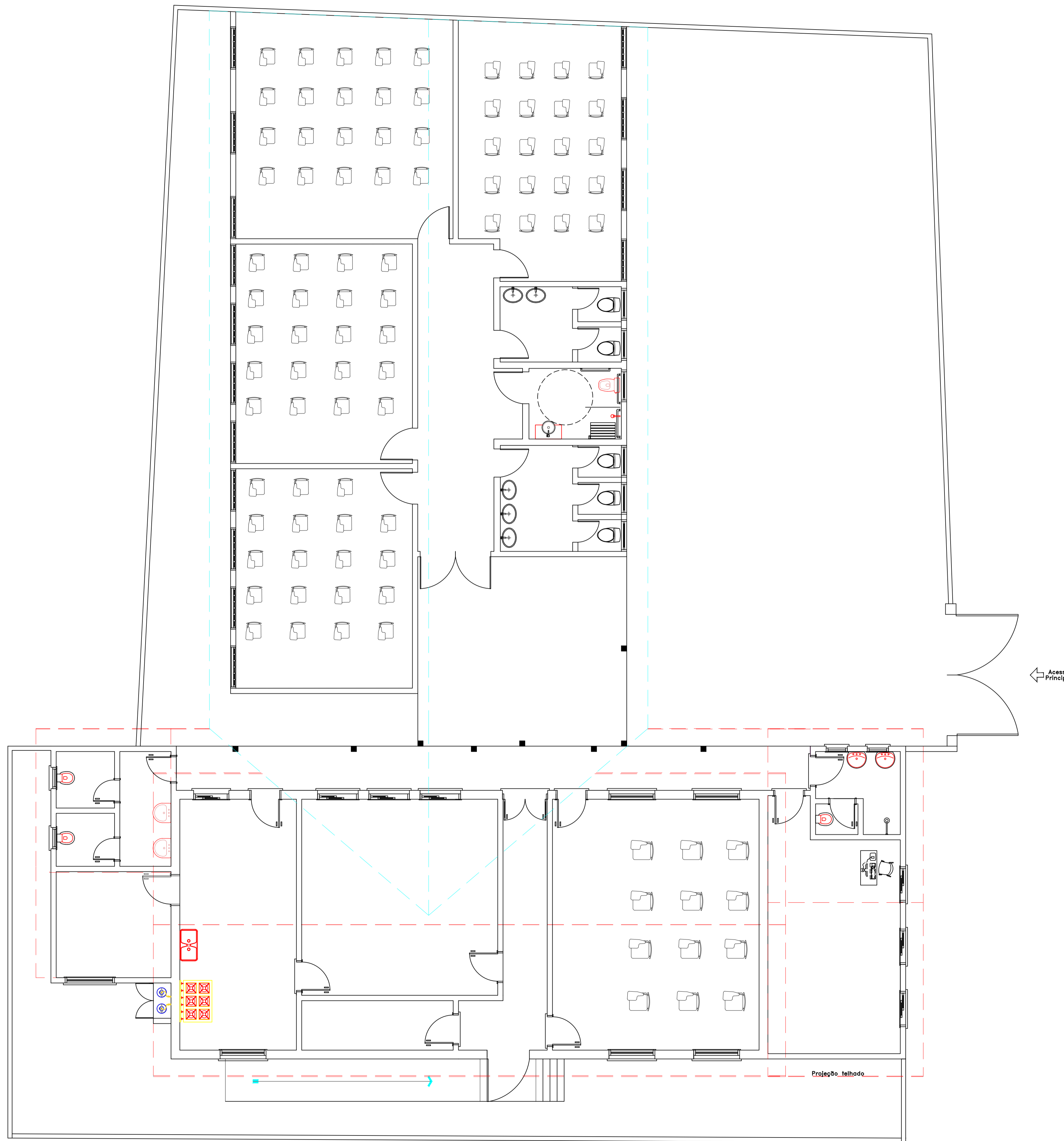
PLANTA BAIXA ARQUITETÔNICA Esc.: 1/75
