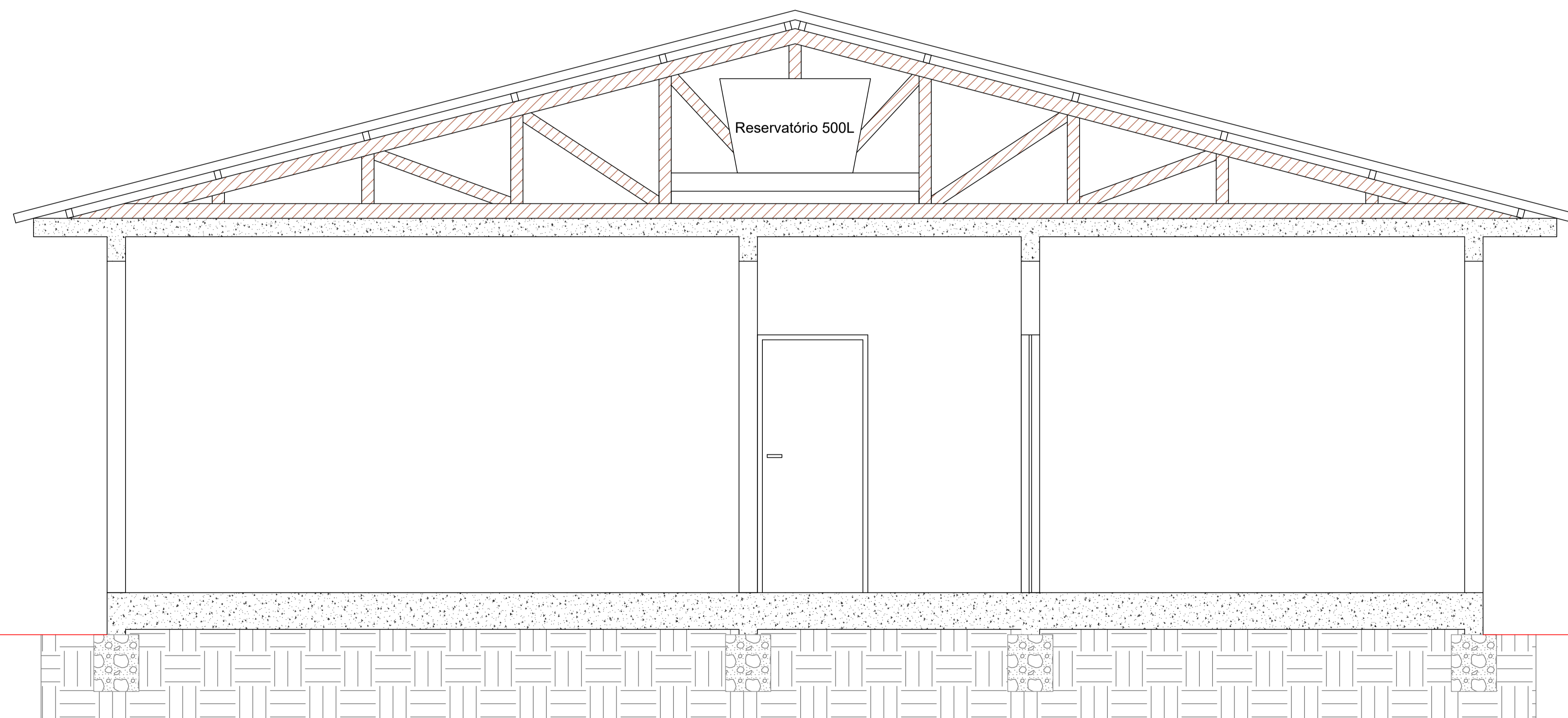
CORTE BB Esc.: 1/20
